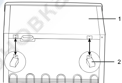
Рисунок Б.2 - Схема крепления упоров до крышки Рисунок Б.2 - Схема крепления упоров к крышке Şəkil B.2 - Dayaqların qarağa bərkidilmə sxemi Бөбө Б.2 - Сахурәвәгә сағрдеғебелди дамағребелди скёбә Б.2-сурет - Тиреишти қақпаққа бекіту схемасы Figura B.2 – Schema fixării de sarac a opritorului B.2-rasm: Tirgaklarni ustki qismga o'rnatish chizmasi.
